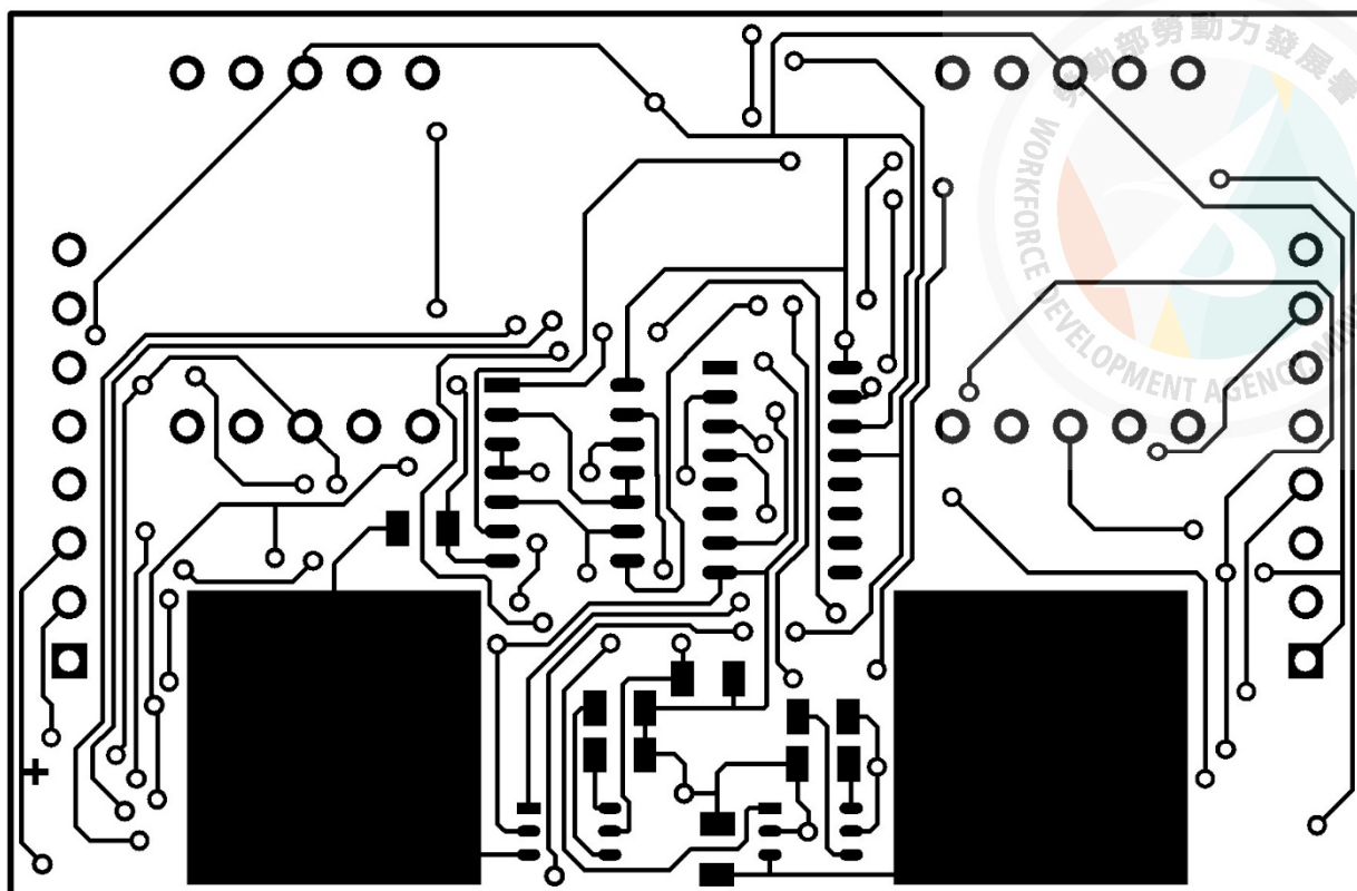
觸控子板電路板正面（Top）佈線圖
