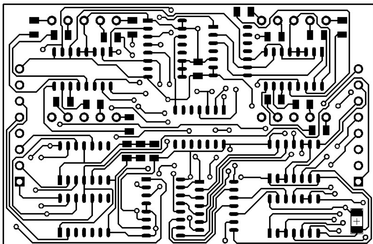
觸控子板電路板反面（Bottom）佈線圖（左右相反）
