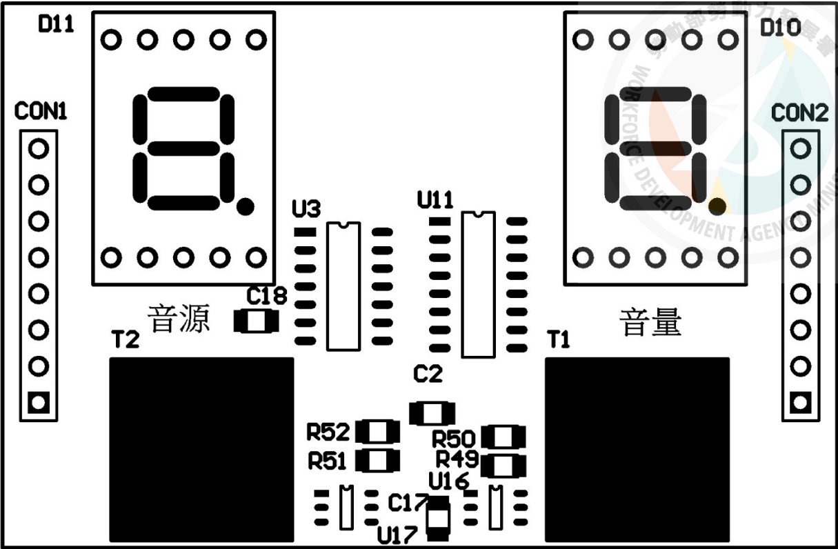
觸控子板電路板正面（Top）元件佈置圖
