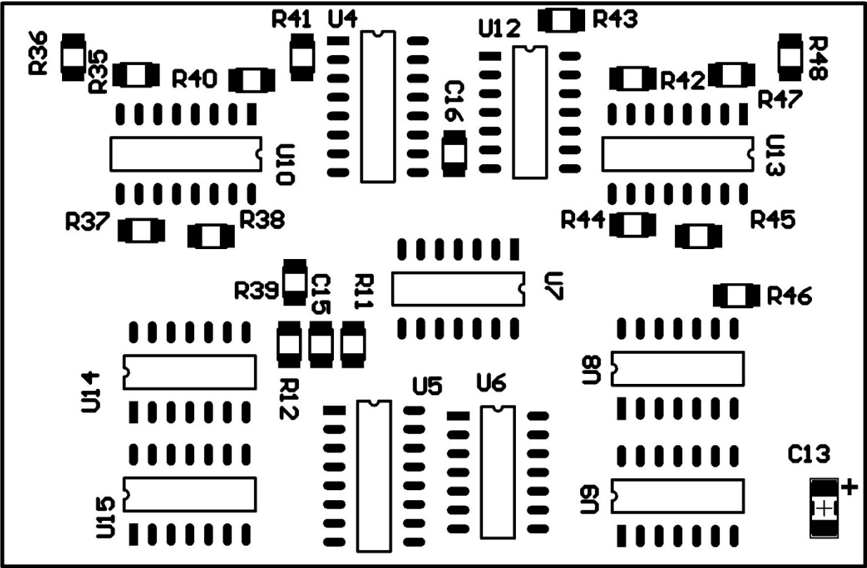
觸控子板電路板反面（Bottom）元件佈置圖（左右相反）
