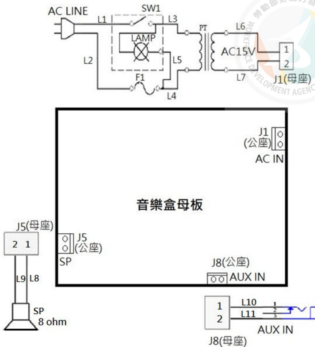
音樂盒連接端子配線圖
