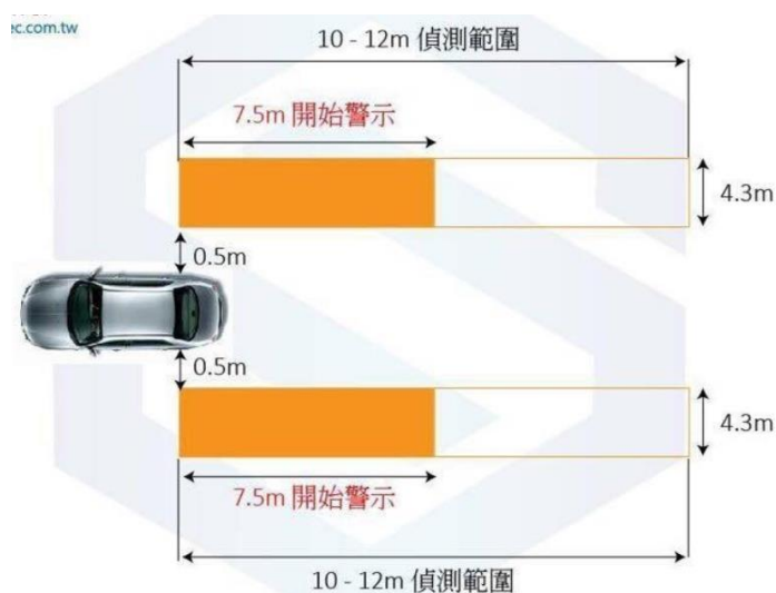
圖 1-1 後方來車可偵測的示意圖(參考興運科技)
