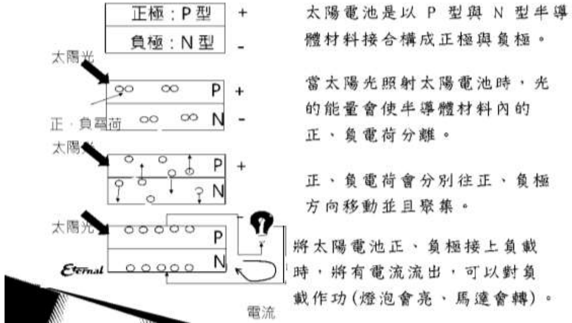
圖 4 太陽能發電原理
