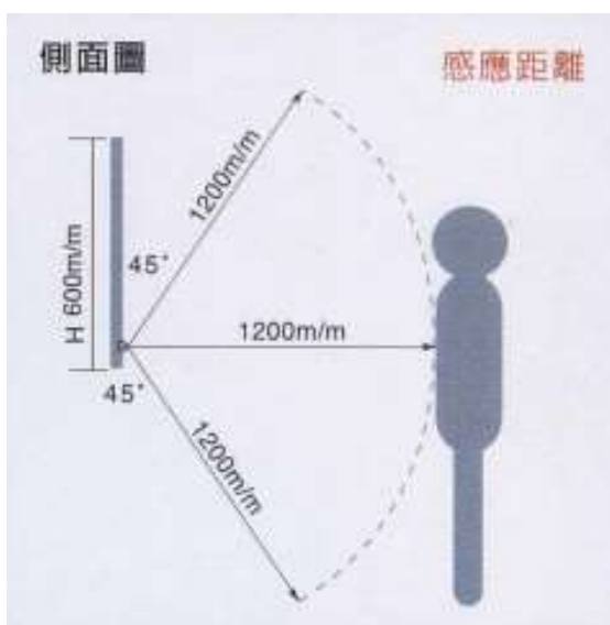
圖 1 原理圖
