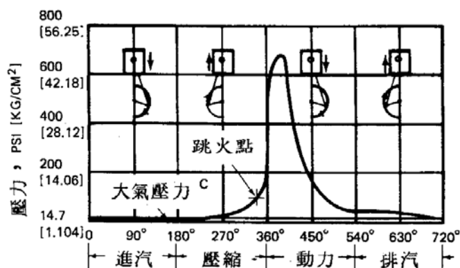
圖十四點火時間的位置
