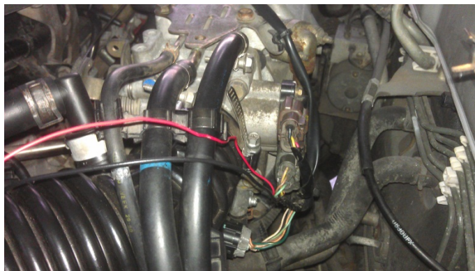
圖十九實車節氣門怠速接點
