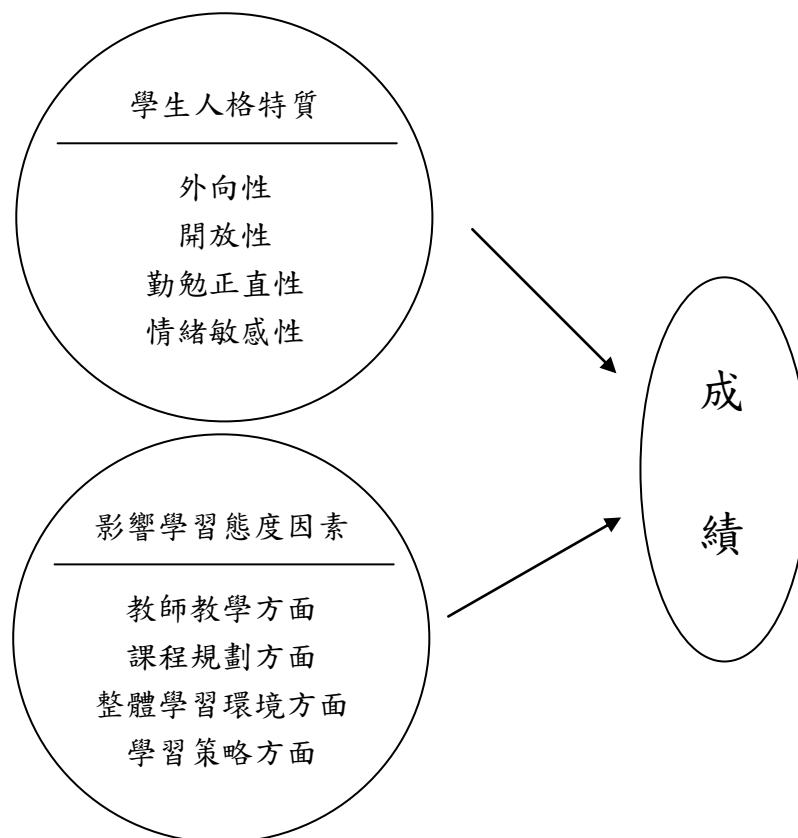
圖 2 研究架構圖
