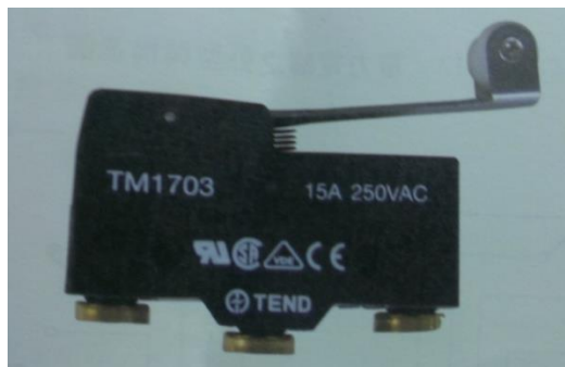
圖七 微動開關
