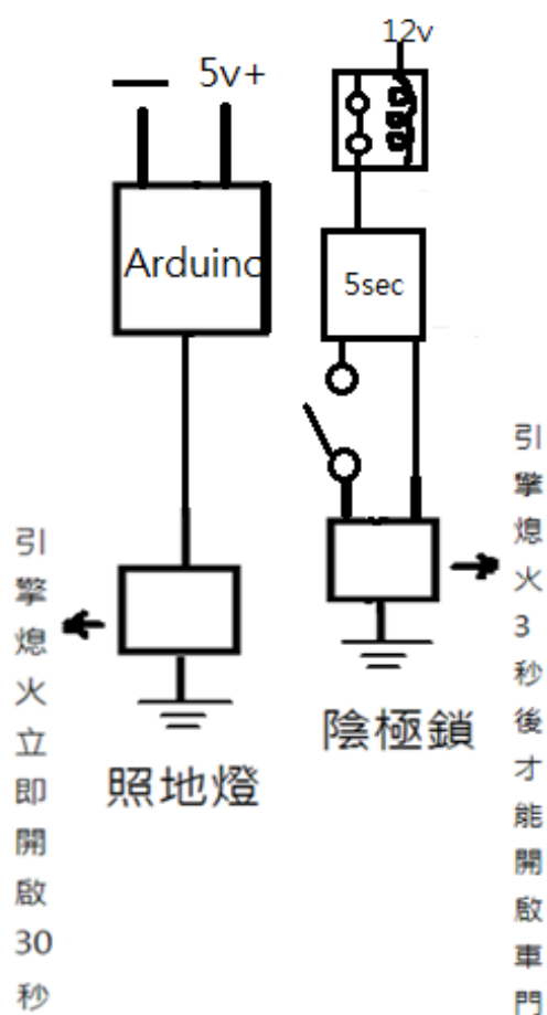
圖 11 警示器電路架構
