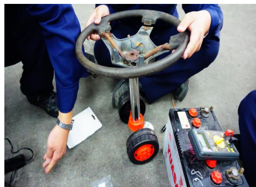
圖22為 模擬轉向機製作完成
