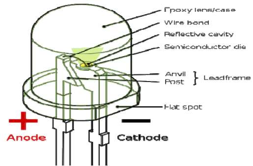
圖(6)發光二極體
