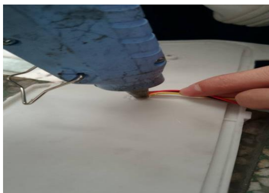
圖6 將熱熔膠補上三角板的空隙
