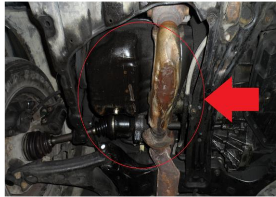
(圖 3-7) 排氣管高溫源與機油殼接近易起火燃燒
