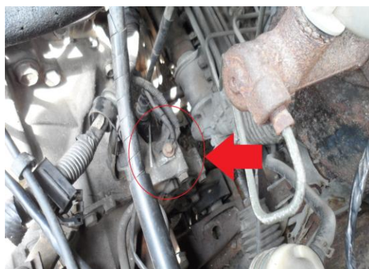
(圖 3-4)電瓶正負極鬆脫容易造成搭鐵產生火花起火燃燒
