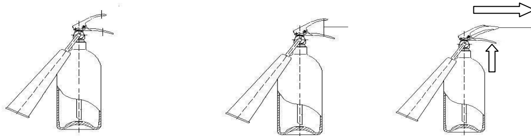
(1) 把滅火器固定引擎室內 (2) 將鋼線穿入把手 (3) 拉動鋼線使其作動
