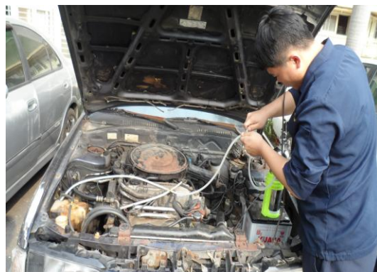
(圖4-9) 將管線長結合滅火器並牽管
