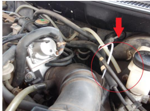
(圖3-15)將管路遷至剎車總泵
