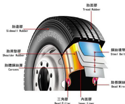
圖 8 輪胎內部介紹
