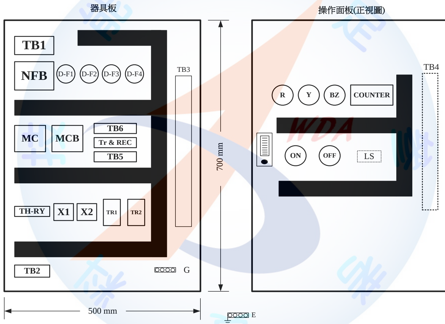
第二站第五題器具位置圖
