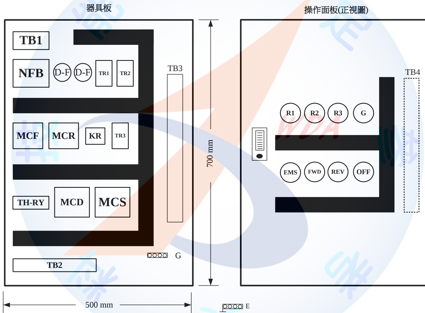
第二站第二題器具位置圖
