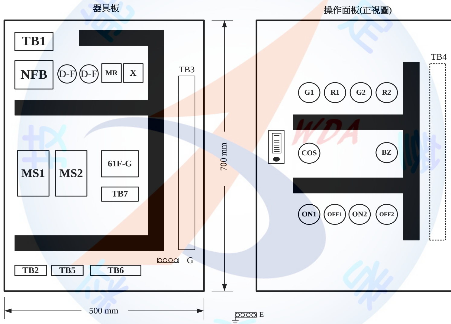
第二站第三題器具位置圖
